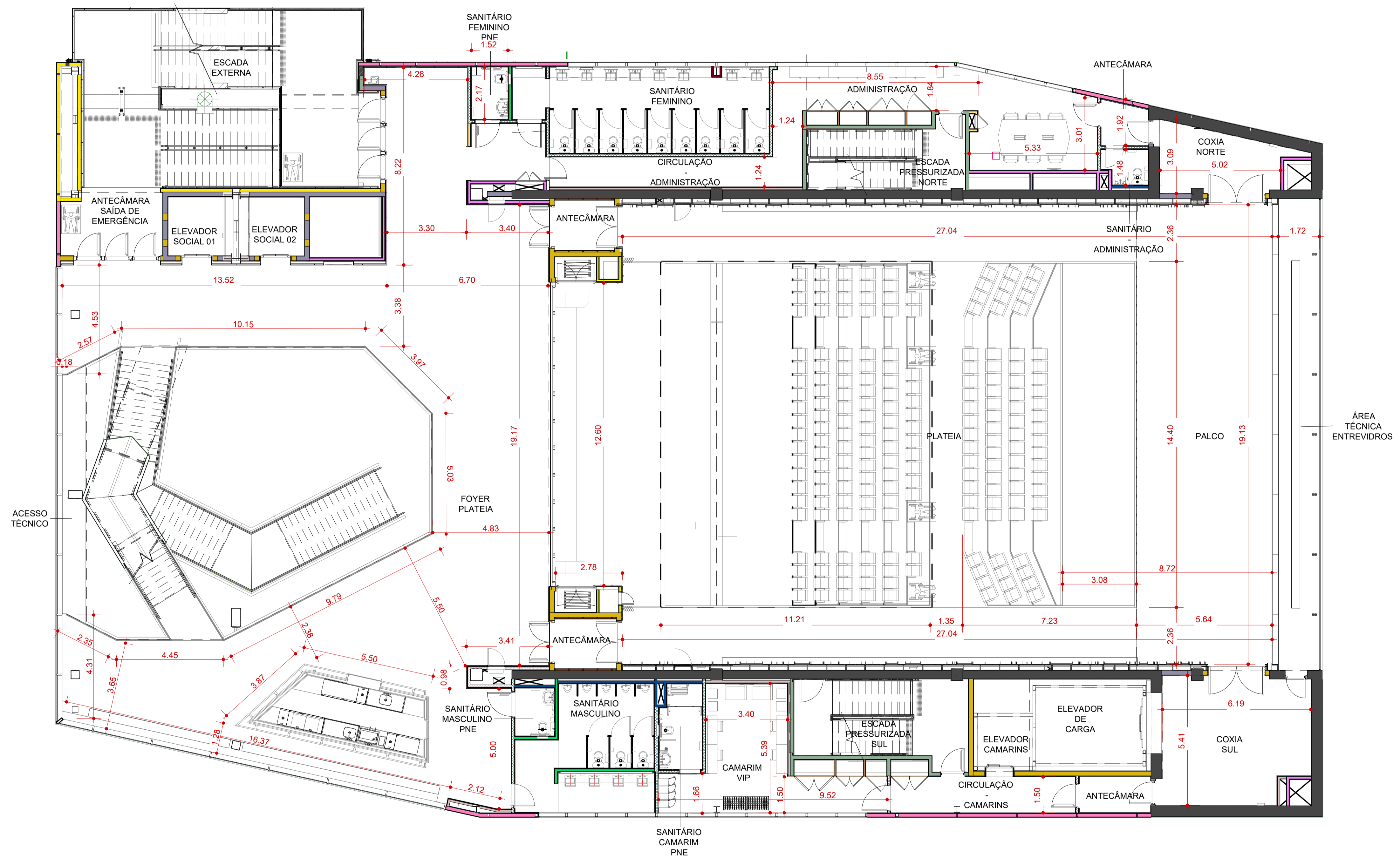
PLANTA BAIXA - NIVEL DA PLATÉIA ESCALA 1:100 MEDIDAS EM METROS (m)
